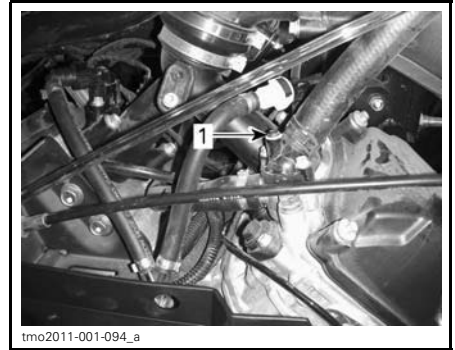
tmo2011-001-094_a TYPIQUE 1. Vis de purge
