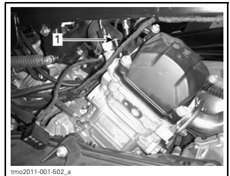
tmo2011-001-502_a 1. Vis de purge du cylindre arrière
