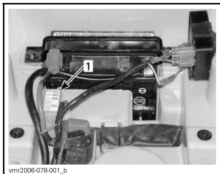
1. Zekeringhouder
