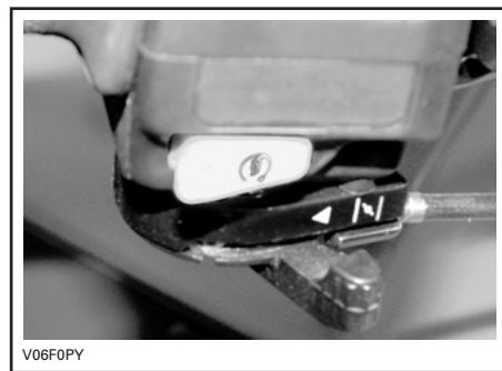
CHOKEHENDEL IN STAND UIT
