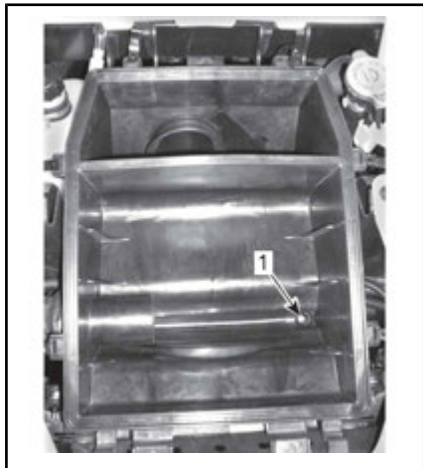
1. Orifício de drenagem
