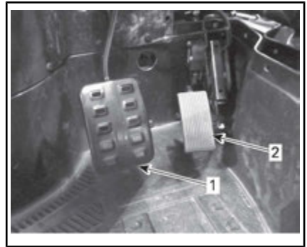
1. Pedal do freio 2. Pedal do acelerador
