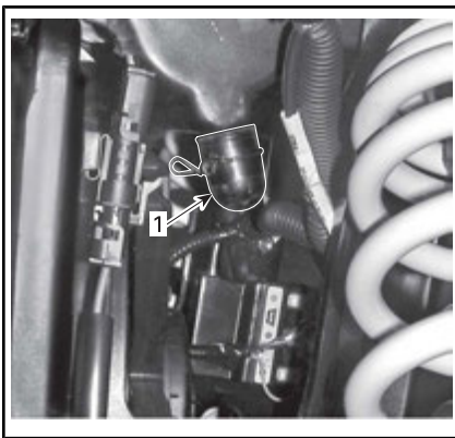
1. Remova o bujão de drenagem para expelir a água
