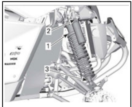
SUSPENSÃO DIANTEIRA — MODELOS DPS X rs E X rs
