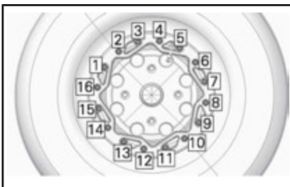
TÍPICO: SECUENCIA DE APRIETE FINAL
