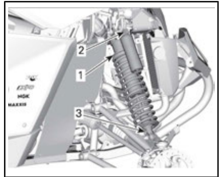
VORDERE AUFHÄNGUNG - ALLE MODELLE AUßER X xc
