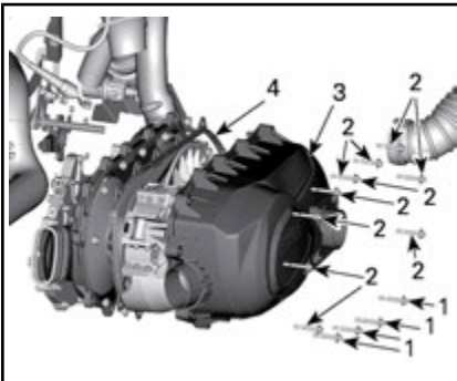
CVT-ABDECKUNG-ANZUGSREIHENFOLGE
