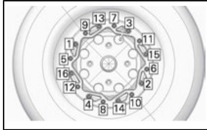
TYPISCH – ANZIEHREIHENFOLGE
