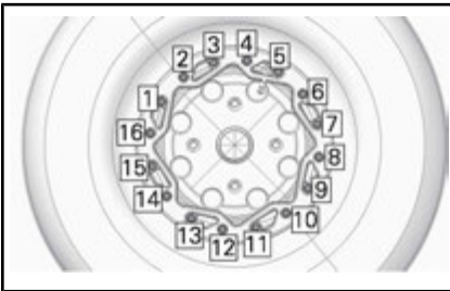
TYPISCH – ENDGÜLTIGE ANZIEHREIHENFOLGE
