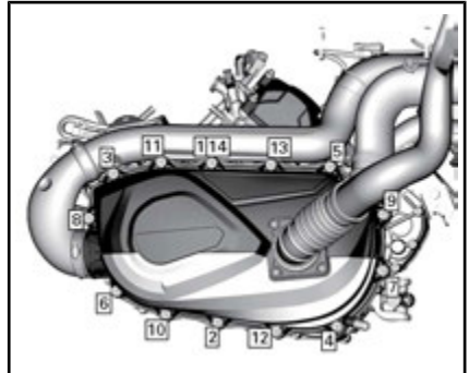
CVT-ABDECKUNG-ANZUGSREIHENFOLGE
