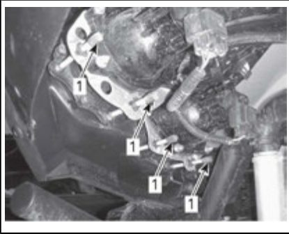
1. Stellschrauben
