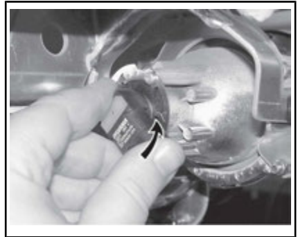
TYPISCH Lampe herausziehen.
