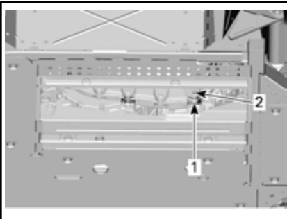
SCHUTZPLATTE ENTFERNT
