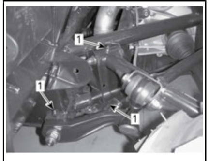
HINTERE AUFHÄNGUNG - TYPISCH
