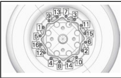
TYPISCH – ANZIEHREIHENFOLGE
