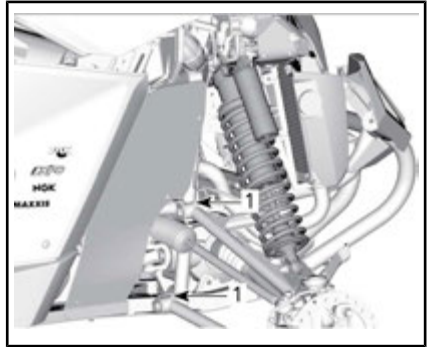
VORDERRADAUFHÄNGUNG - TYPISCH
