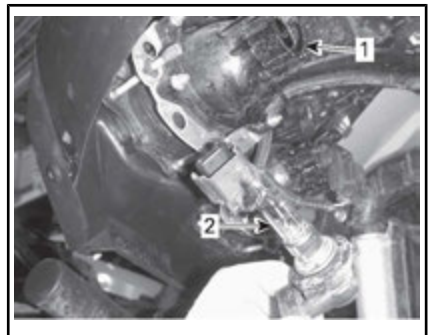
1. Glühlampenfassung 2. Glühlampe
