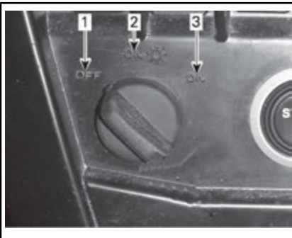
TENNINGSBRYTERENS POSISJONER
