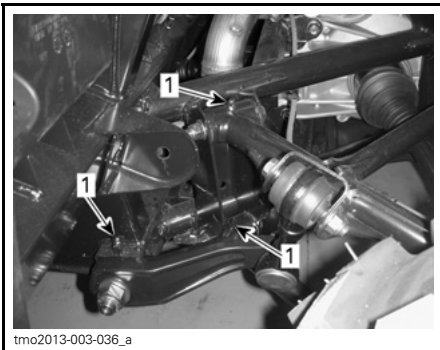
BAKFJÄDRING - TYPBILD
