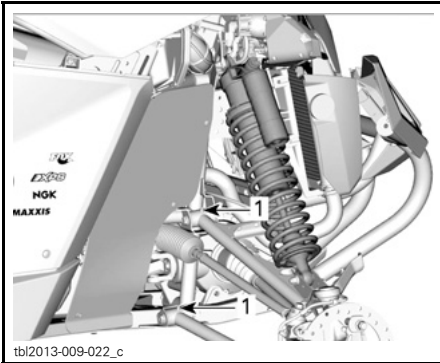
FRAMFJÄDRING - TYPBILD
