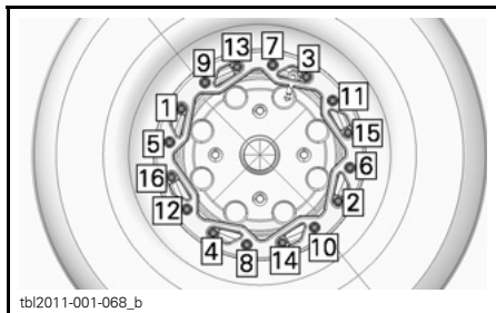
TYPBILD - ÅTDRAGNINGSSSEKVENNS
