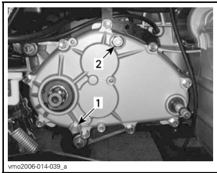
1. Dreneringsplugg for girboks
