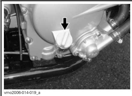
PEILESTAV – HØYRE SIDE AV MOTOREN
