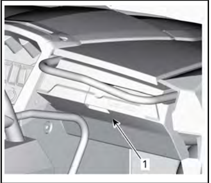
1. Vergrendeling handschoenvak
