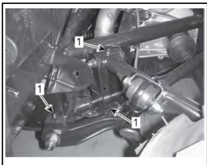
SUSPENSÃO TRASEIRA - TÍPICO
