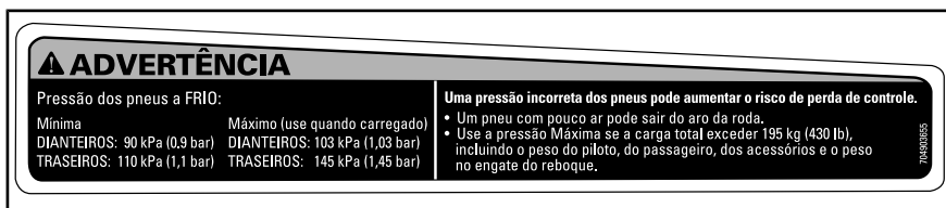
ETIQUETA 9 - FORA DA AMÉRICA DO NORTE
