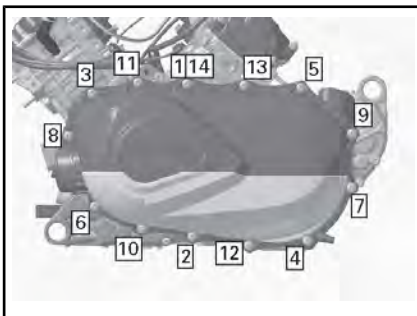
SEQUÊNCIA DE APERTO DA TAMPA DA CVT
