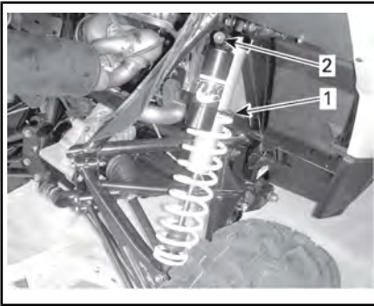
SUSPENSIÓN TRASERA, MODELOS ESTÁNDAR
