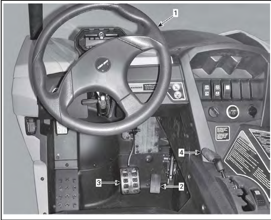
TÍPICO: MANDOS PRINCIPALES
