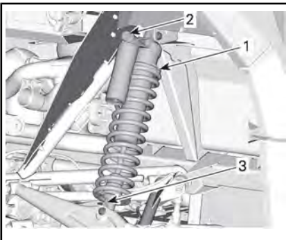
SUSPENSIÓN TRASERA, MODELOS XrsRS
