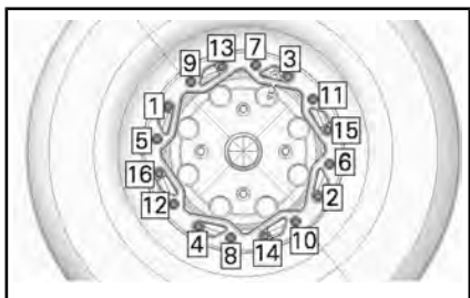
TÍPICO: SECUENCIA DE APRIETE
