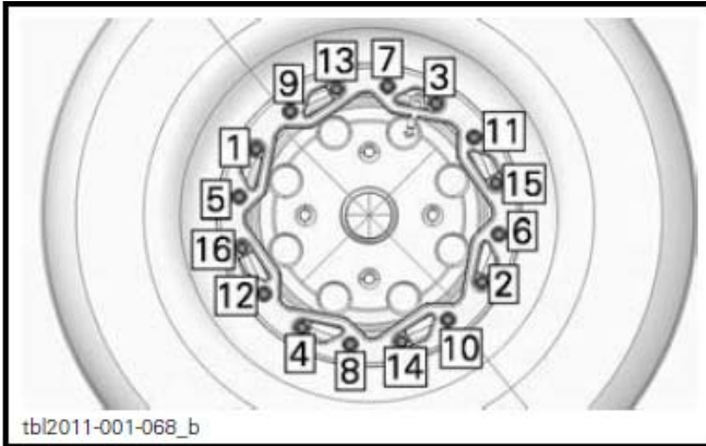
典型图示 - 收紧次序
