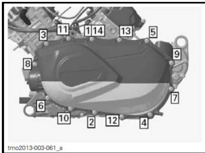
tmo2013-003-061_a 无级变速箱盖收紧次序
