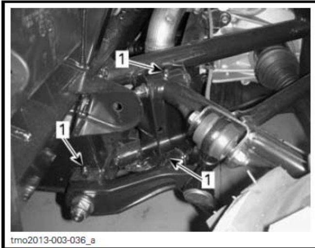
后悬架 - 典型图示
