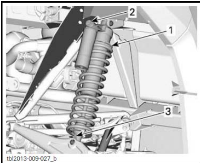
后悬架 – X rs 型号
