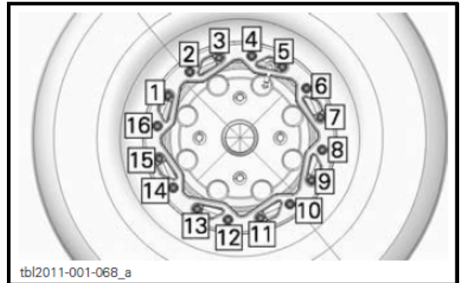
典型图示 - 最后收紧次序
