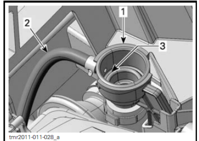
1. 冷却系统添加转接器 2. 胀溢水箱软管 3. 冷却系统全满液位（压力盖座）
