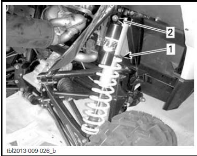
后悬架 – 标准型号
