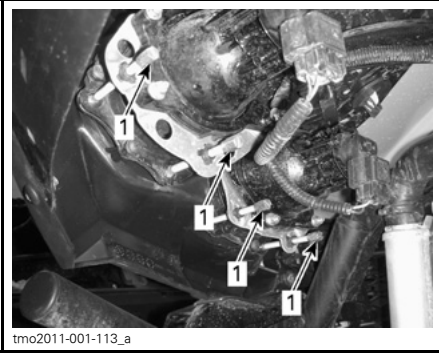
1. Justerings-skruer
