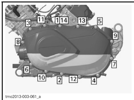
TILTREKKINGSREKKEFØLGE FOR CVT-DEKSEL
