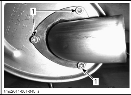
1. Borgschroeven
