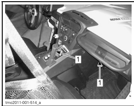
1. Handgrepen passagier
