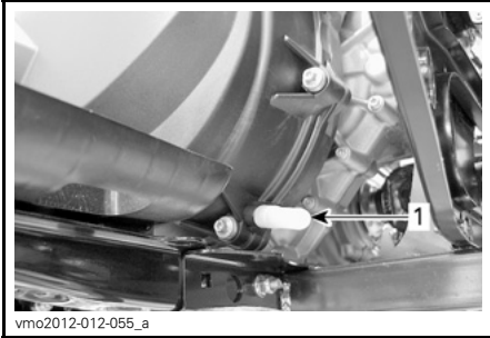
1. CVT-aftap
