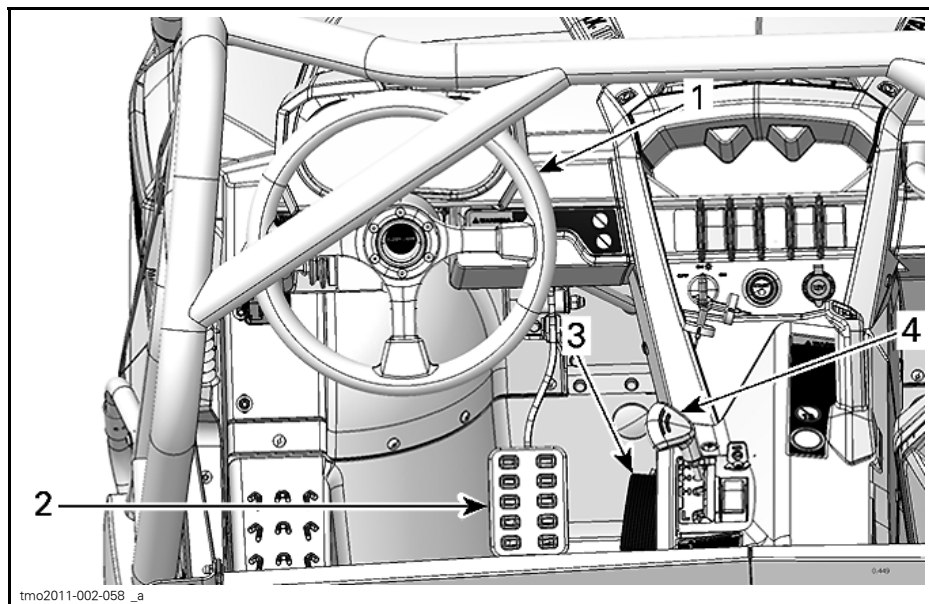
PRIMAIRE BESTURINGSELEMENTEN
