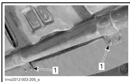
BRIDES AVANT DE LA VISIÈRE SPORT
