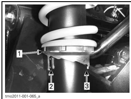
TYPIQUE 1. Tourner les cames de réglage 2. Réglage souple 3. Réglage ferme
