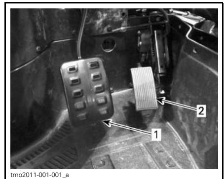
1. Pédale de frein 2. Pédale d'accélérateur
