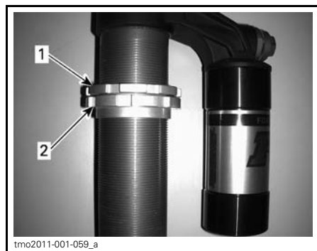
TYPIQUE - RESSORT NON ILLUSTRÉ 1. Desserrer l'anneau de verrouillage supérieur 2. Tourner l'anneau de réglage en conséquence
