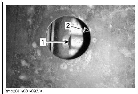
1. Tapón de drenaje de aceite 2. Apertura del protector de bajos
