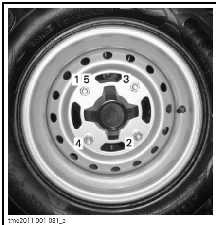
SECUENCIA DE APRIETE
