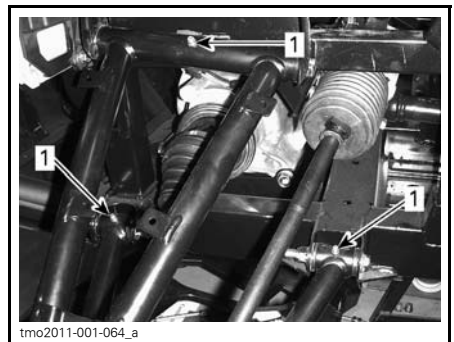
SUSPENSIÓN DELANTERA - TÍPICO 1. Puntos de engrase
