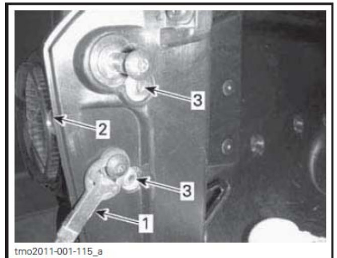
1. 后挡板钢索 2. 尾灯 3. 固定螺丝
