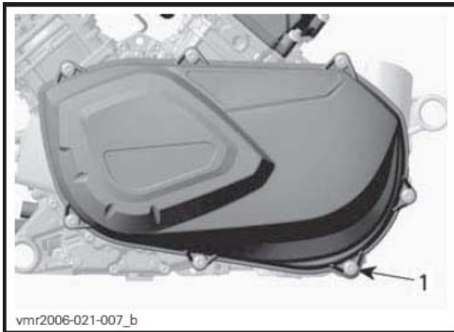
1. 无段变速箱盖排放螺丝
