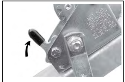
RÉGLER LE TREUIL À LA POSITION D'ENROULEMENT
