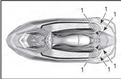
1. Självgängande skruvar
