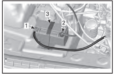
CARROSSERIE CENTRALE RETIRÉE À DES FINS DE CLARTÉ
