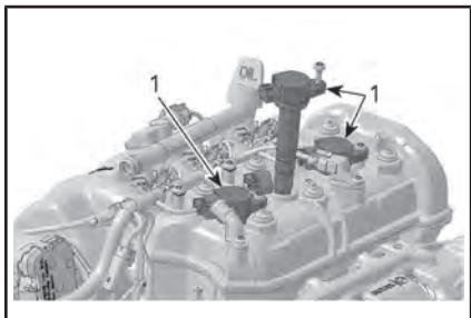
1. Bobines d'allumage
