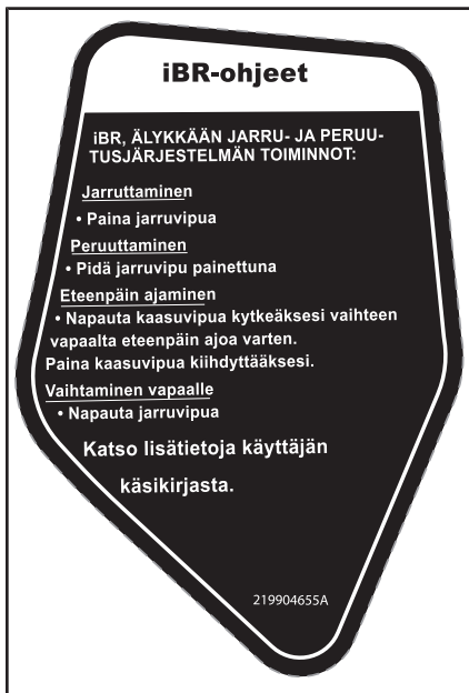
KILPI 13 - SIJAITSEE KONSTOLISSA - MALLIT, JOISSA iBR
