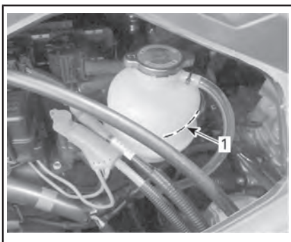
1. 冷却液液位标记
