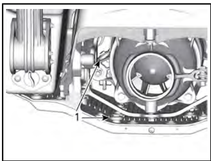
1. Anodi sacrificali
