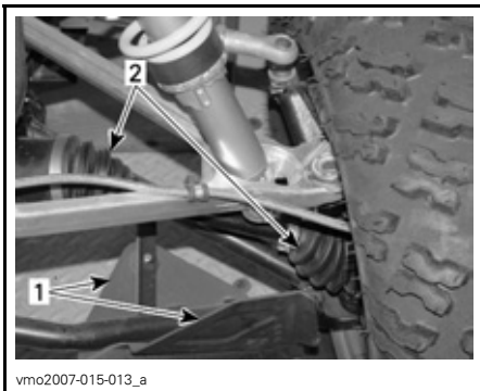
VOORKANT VOERTUIG 1. Beschermer aandrijfjas 2. Manchetten aandrijfjas
