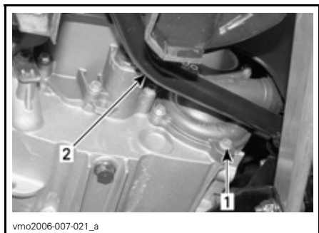
vmo2006-007-021_a 1. Koelvloeistof-aftapplug 2. Rempedaal
