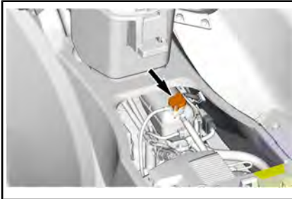
Etiqueta del silenciador de la entrada de aire
