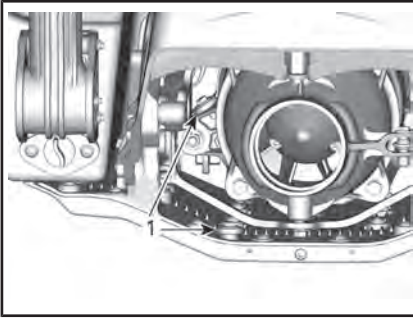
1. Ânodos sacrificiais
