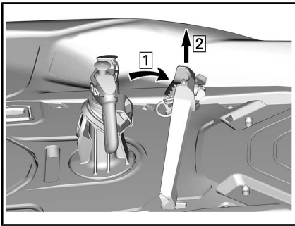
1. Kippträger 2. Hebeträger
