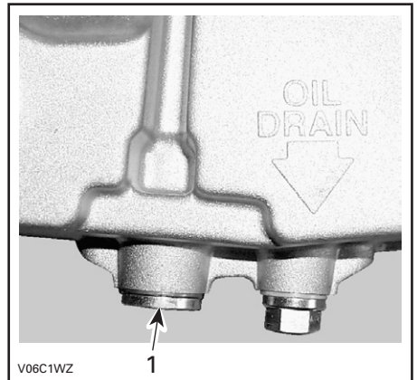
1. Tapón del depurador de aceite
