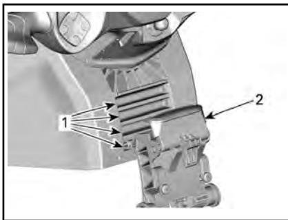
STUURKOLOMVERGRENDLING BEVESTIGD
