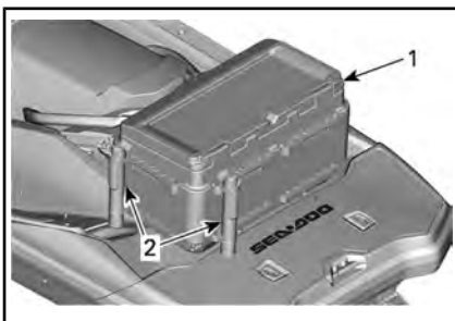
1. Koeler 2. Vishengelhouder
