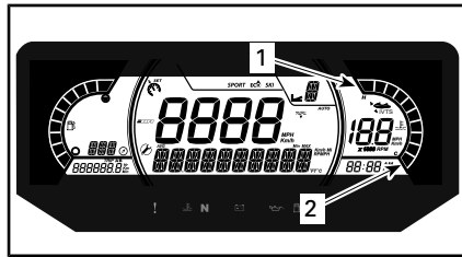
INFORMATIECENTRUM — VTS-POSITIE-INDICATOR
