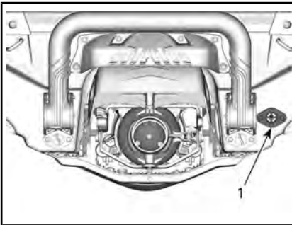
1. Wassereinlassstutzen
