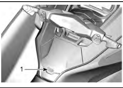
1. Deckelbefestigung
