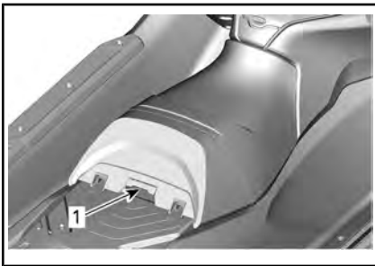
1. Verriegelungshebel
