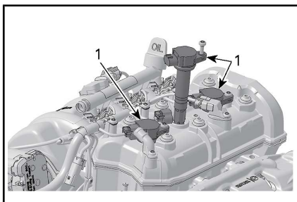
1. Tändspolar
