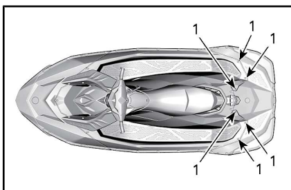
1. Självgående skruvar
