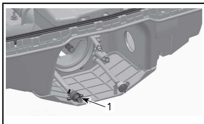
JETPUMPSMUNSTYCKE BORTTAGET FÖR TYDLIGHETENS SKULL
