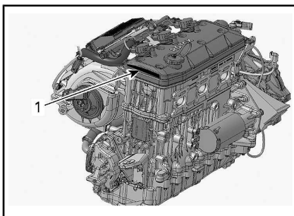
1. Número de Identificação do Motor (EIN)
