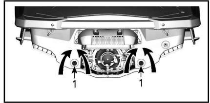
LOCALIZAÇÃO DOS BUJÕES DE DRENAGEM DO BOJO
