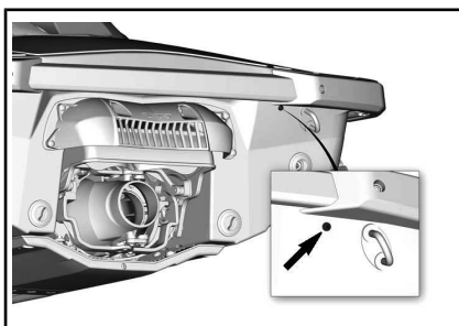
CONEXÃO DE TRANSBORDAMENTO DO INTERCOOLER
