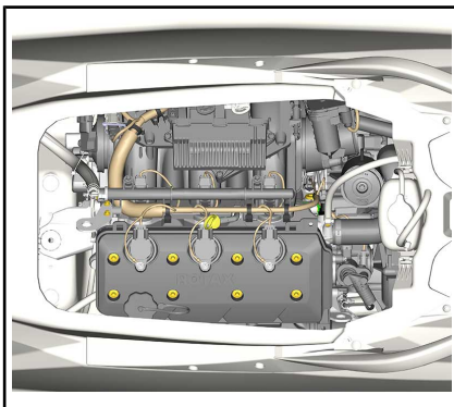
发动机舱，已拆下座椅
