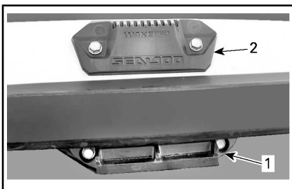
尾波滑水板齿条的固定架
