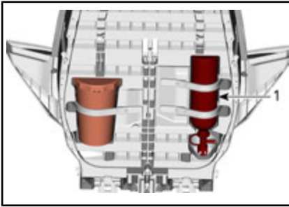
1. 消火器
