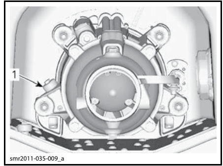
1. Расположение защитных анодов.
