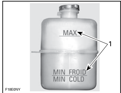
ТИПОВОЙ ВАРИАНТ — РАСШИРИТЕЛЬНЫЙ БАЧОК
