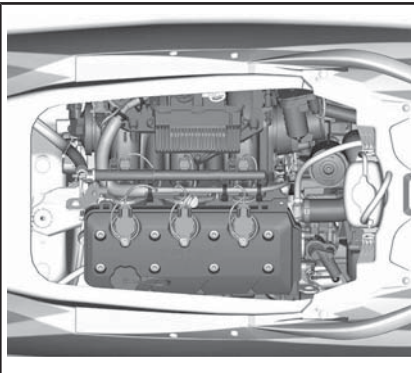
COMPARTIMENTO DEL MOTOR, ASIENTO RETIRADO
