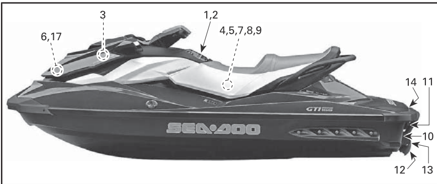
UBICACIÓN DE LAS ETIQUETAS DE SEGURIDAD EN LA MOTO ACUÁTICA - MODELOS GTI
