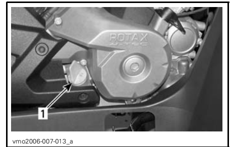
1. Jauge de niveau d'huile
