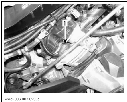
vm02006-007-029_a CÔTÉ DROIT — CYLINDRE ARRIÈRE 1. Bougie
