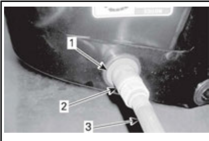
ADAPTADOR DE MANGUERA DE CONEXIÓN RÁPIDA
