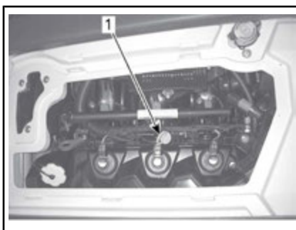
TYPISCH - 260ER-MOTOREN
