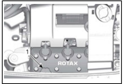
TYPISCH - ALLE MODELLE AUßER BEI 260 MOTOREN
