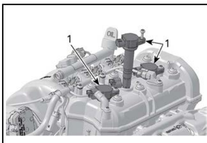
1. Bobinas de encendido
