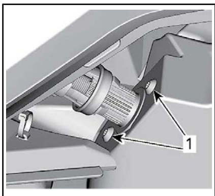
1. Tornillos del sistema de cables
