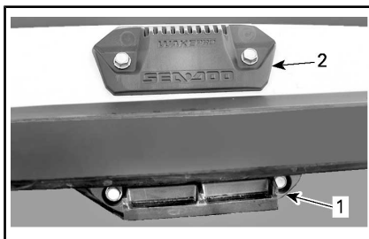
SUPORTES PARA O RACK DE WAKEBOARD
