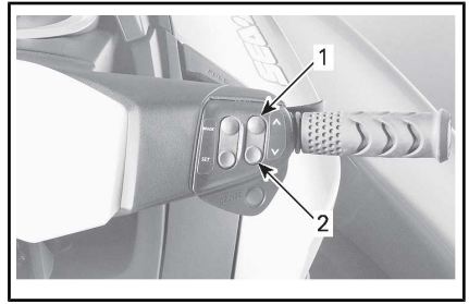
TÍPICO - AJUSTE DE LA POSICIÓN DE PUNTO MUERTO DEL iBR
