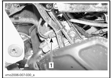
LINKERKANT — VOORSTE CILINDER 1. Bougie
