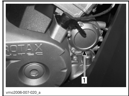
1. Oliefilterdeksel
