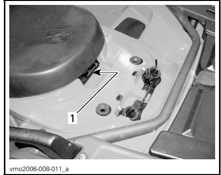
1. Vergrendeling zitting
