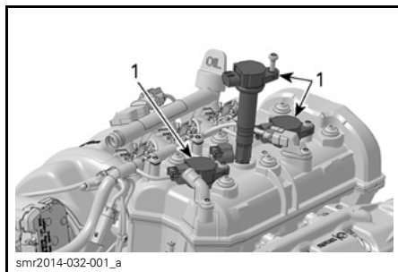
1. Tändspolar
