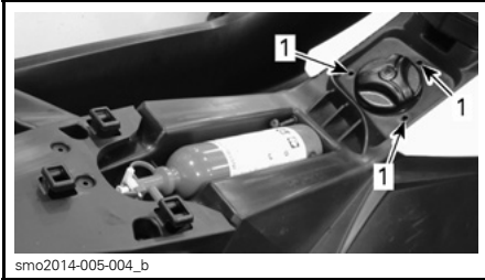
1. Skruvar
