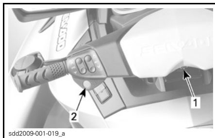
TYPEBILDE 1. Motorstoppbryter 2. START/STOPP-knapp
