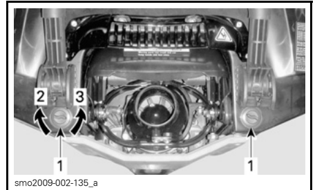
TYPEBILDE – PLASSERING AV DRENERINGSPLUGGER FOR BUNNVANN
