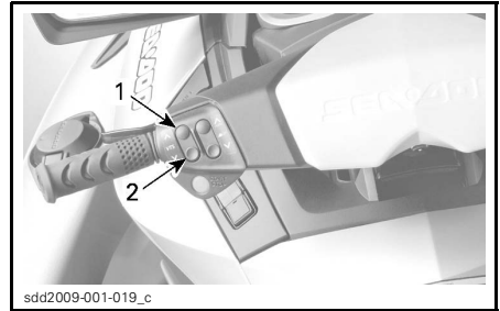
TYPIQUE - BOUTON DE COMMANDE VTS
