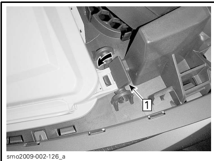
Étape 1: Pousser les fermoirs vers le bas pour immobiliser le bac
