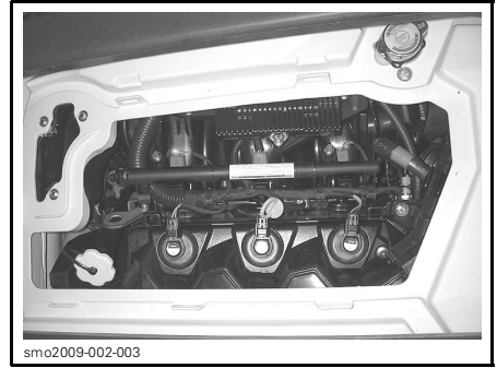
smo2009-002-003 BOÎTE DE VENTILATION RETIRÉE
