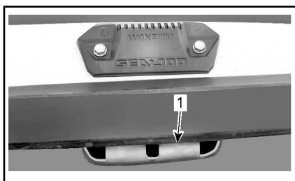
HALTEBESCHLÄGE FÜR WAKEBOARD-HALTERUNG
