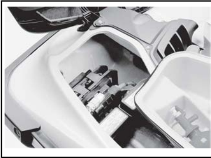
ZUGRIFF AUF BATTERIE UND SICHERUNG - RECHTER VERSTAUBEHÄLTER ENTFERNT
