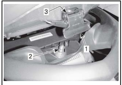
TYPISCH - SCHLIEßMECHANISMUS DES SITZES
