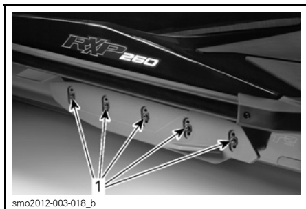
1. Selvklebende skruer
