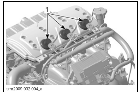
1. Forsegling riktig plassert
