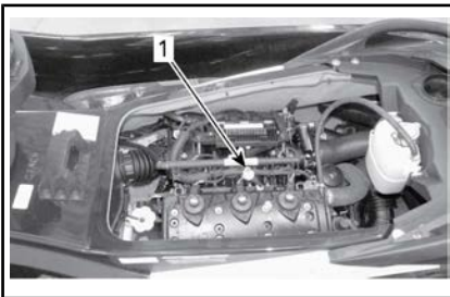
1. Ubicazione dell'astina dell'olio
