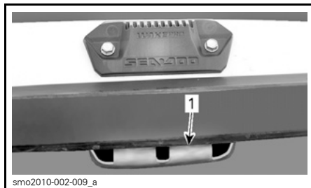
1. Festet del av stativet i nedre brakett
